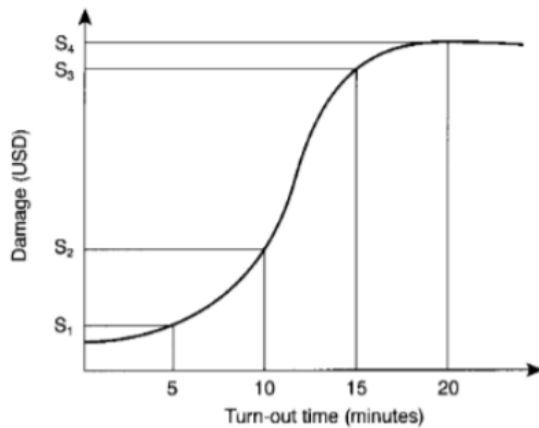
Figur 8: Sammenheng mellom utfall fra en brann og brannvesenets responstid. Kilde: Mattson og Juås (1997)
